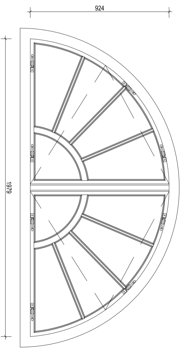
Okno zewnętrzne (przekrój od strony pomieszczenia)
